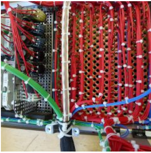
Adapter-Verdrahtung
